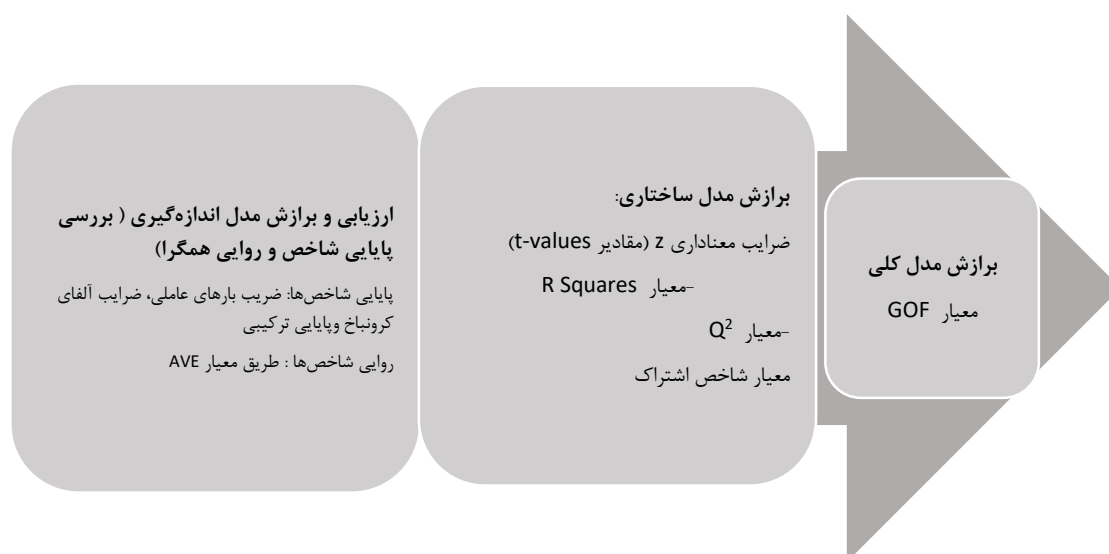
شکل (۱) روش ارزیابی مدل معادلات ساختاری (اقتباس از Jony et al., 2020: 222).
