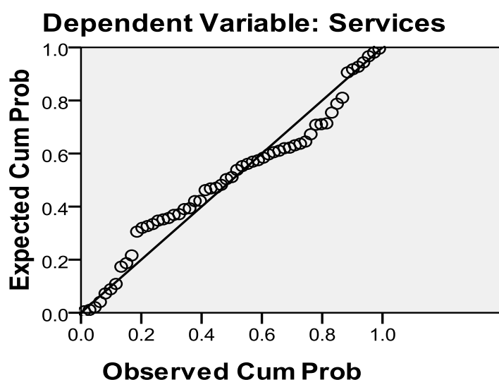
شکل شماره (۴): نمودار خط نرمال باقی مانده‌های مدل رگرسیونی
