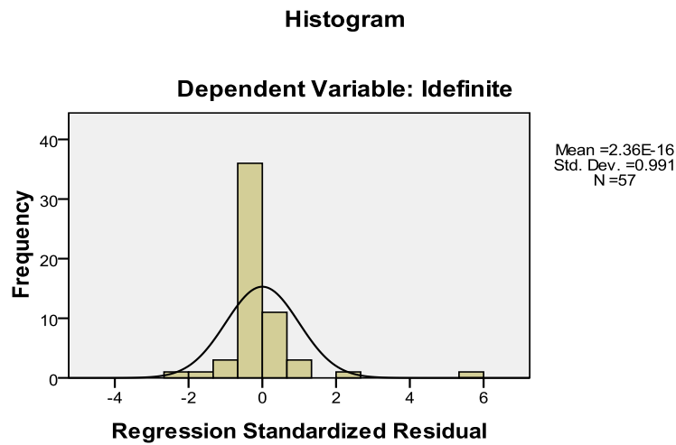
شکل شماره (۵): هیستوگرام متغیر وابسته توزیع داده‌ها برای آماره‌های باقی مانده
